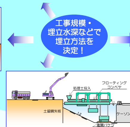
底開式バケット方式
