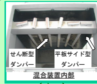
せん断型 ダンパー 混合装置内部 平板サイド型 ダンパー
