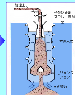
ジャンクション シュート方式
