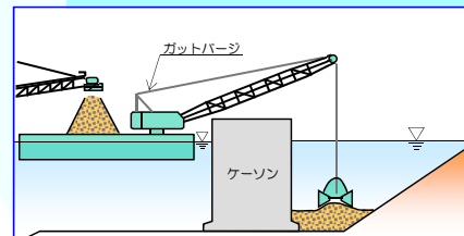
クラムシェル バケット方式
