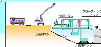
底開式バケット方式
